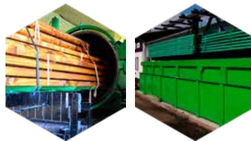
Vakuo-tlaková impregnace Impregnace v máčecí vaně
